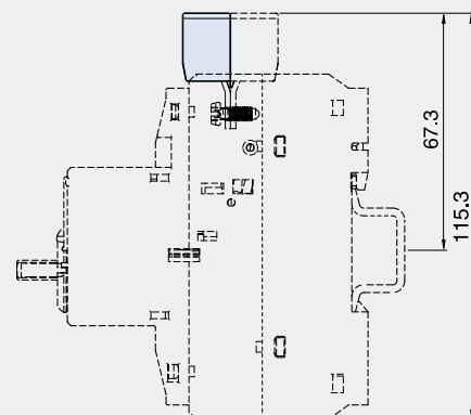
MMS-32H/32HI+PB-322(2 Terminal) PB-322(2 Terminal), PB-323(3 Terminal)
