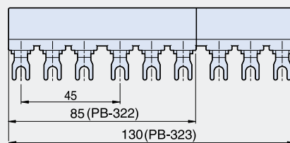
MMS-32H/32HI+PB-322(2 Terminal) PB-322(2 Terminal), PB-323(3 Terminal)
